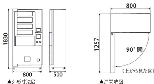
▲外形寸法図
