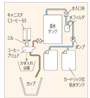
▲原理図
